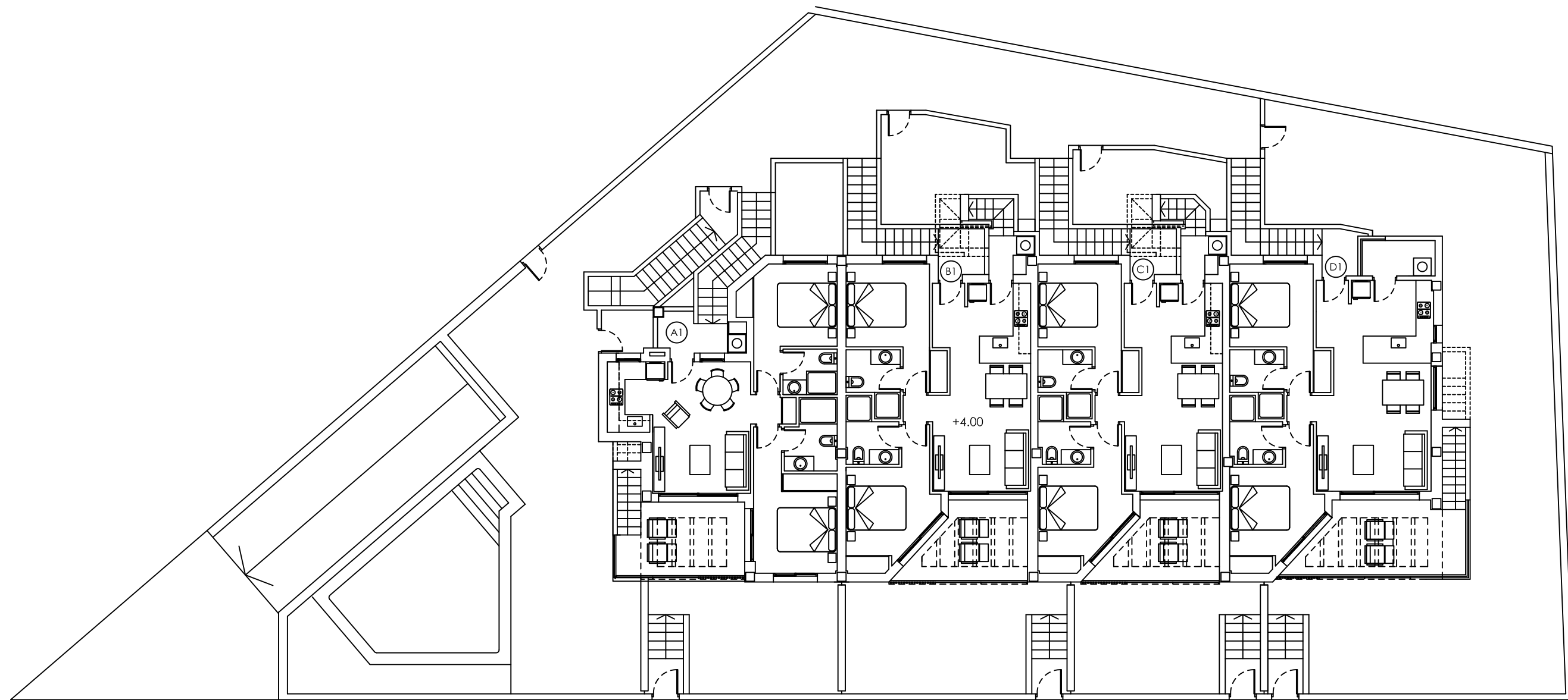
PLANTA ALTA
